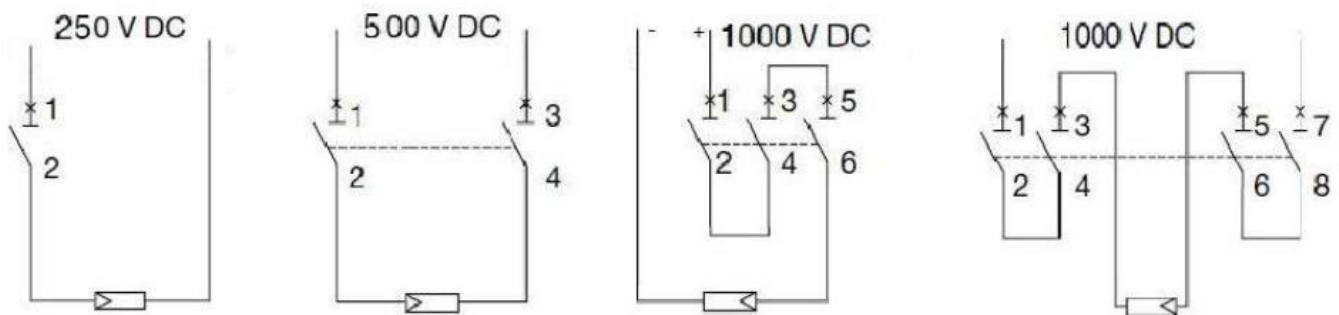
不接地系统
